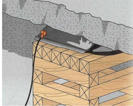
(그림 2-7) 받침목을 이용한다.
