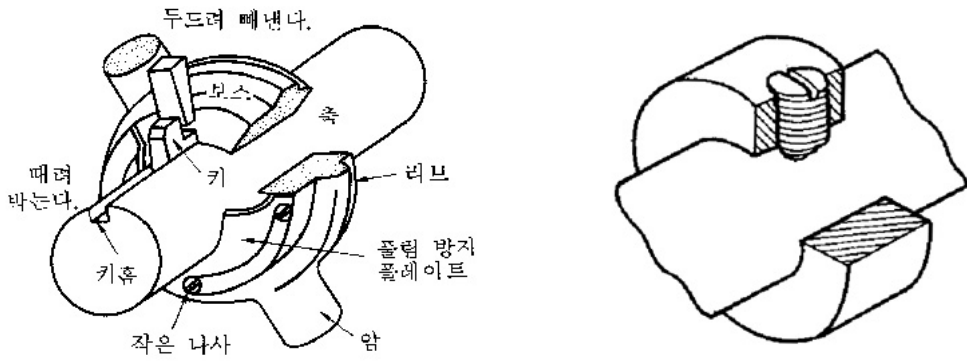
(그림 5-10) 키와 나사로 고정된 축의 분해방법
