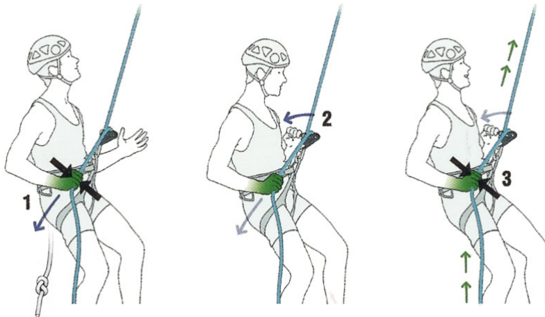
(그림 3-66) GriGri를 사용할 때 아래 손은 항상 로프를 잡고 있어야 한다.
