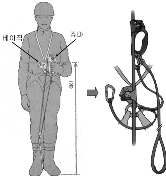
(그림 3-84) 슬링의 길이를 적절히 조정한다.
