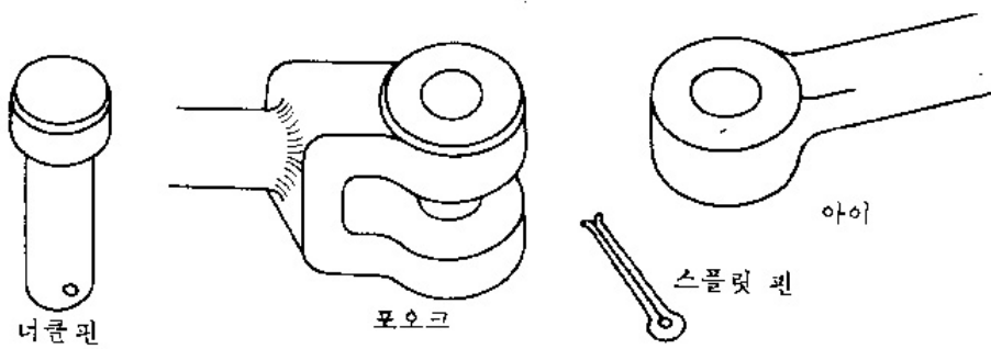
(그림 5-13) 링크로 연결된 부분은 먼저 스플릿 핀을 제거하고 너클핀을 뺀다.
