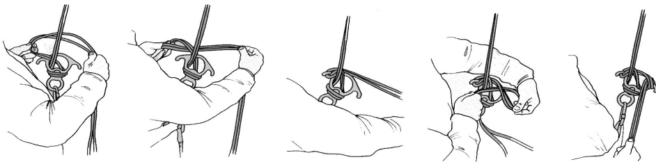
(그림 3-80) 구조용 하강기를 고정하는 방법
