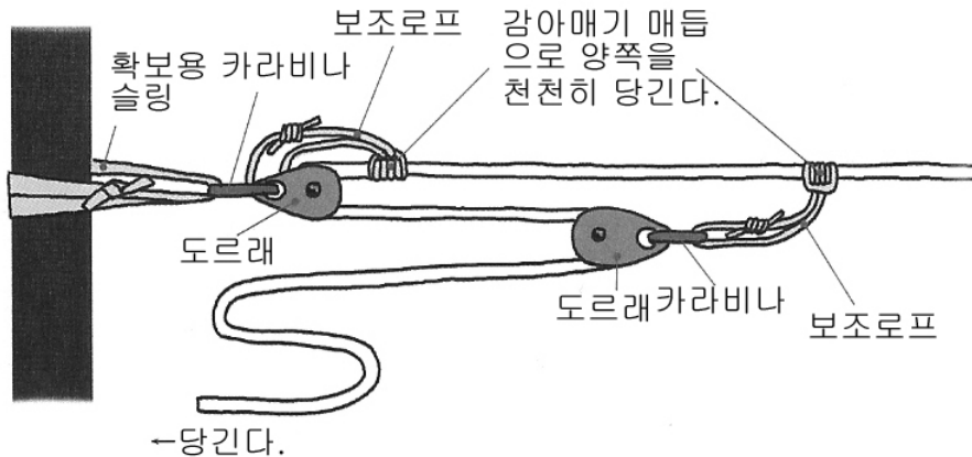
(그림 3-60) Z자형 도르래 배치법을 응용한 로프 연장법
