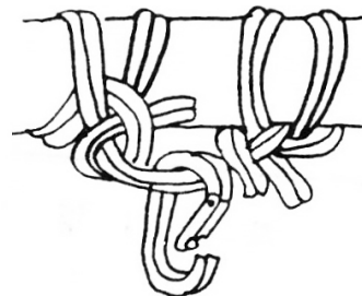
(그림 3-47) 지점의 설치 예시 (기둥에 말뚝매듭을 하고 카리비나를 끼웠다. 매듭의 끝 부분은 풀리지 않도록 움매듭으로 확실히 고정한다.)
