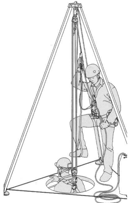
(그림 2-4) 맨홀 구조기구
