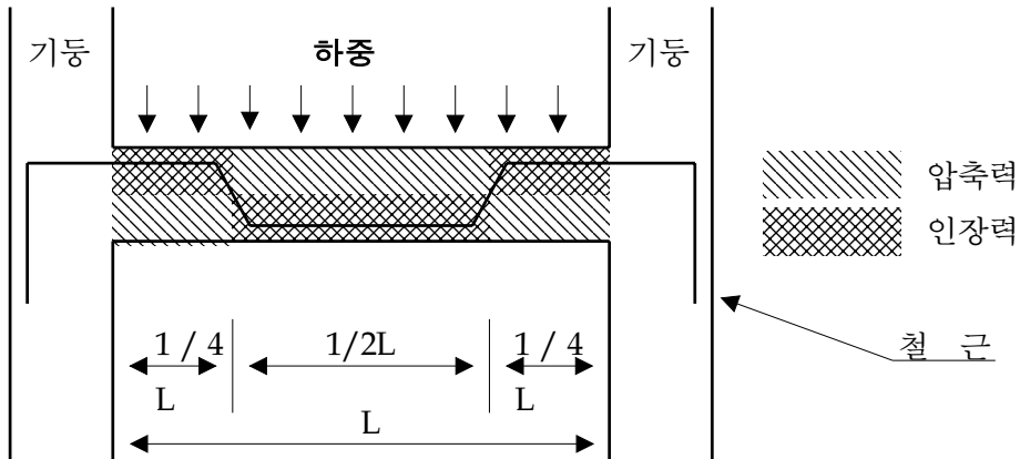
(그림 5-86) 보의 응력 분포
