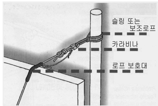
(그림 3-50) 현수로프의 간접 고정
