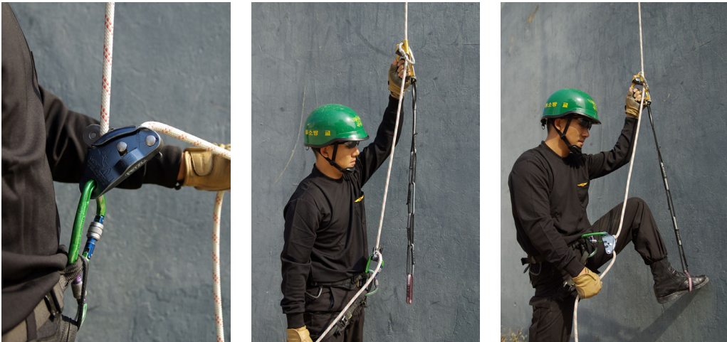
(그림 3-87) 그리그리와 jumal에 현수로프를 삽입한다. 슬링의 고리에 발을 넣고 힘차게 일어선다.
