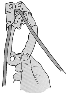
(그림 3-86) 로프가 이탈하지 않도록 카라비나를 끼워둔다.
