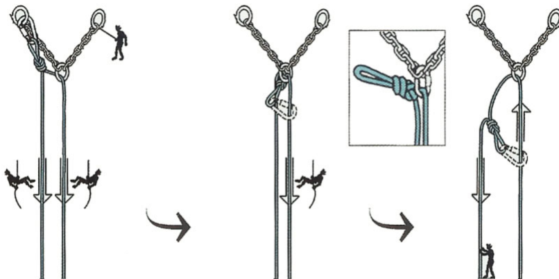
(그림 3-53) 회수로프 설치방법
