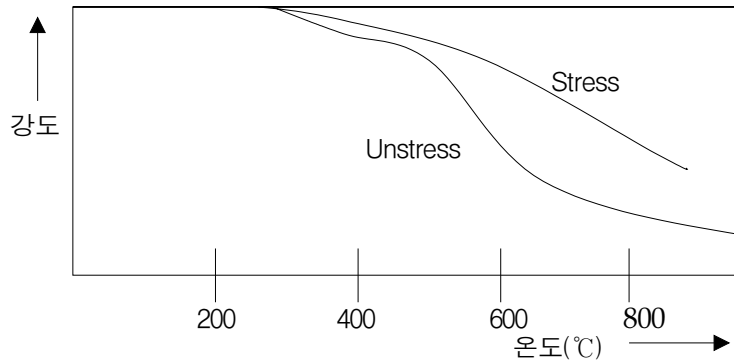
(그림 5-87) 콘크리트의 온도변화에 따른 강도 변화
