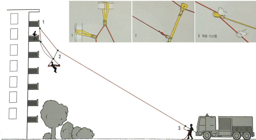
(그림 4-16) 경사하강으로 구조하기
