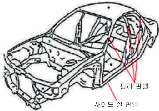
(그림 5-42) 필라 판넬의 위치
