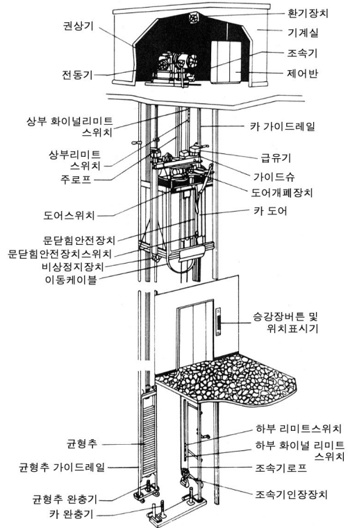
(그림 5-103) 엘리베이터의 구조
