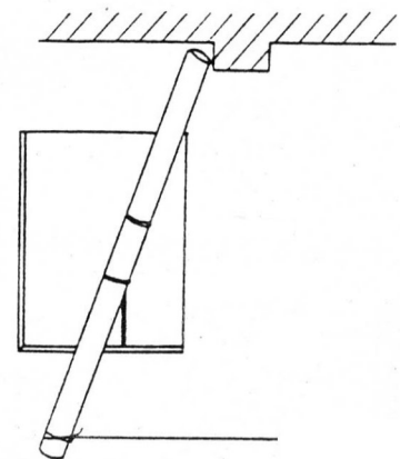
(그림 3-41) 창문을 활용한 확보점 만들기의 예
