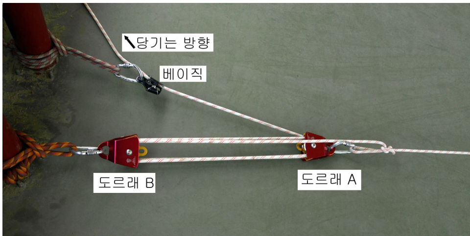
(그림 3-61) 2단도르래를 이용한 로프 연장 방법
