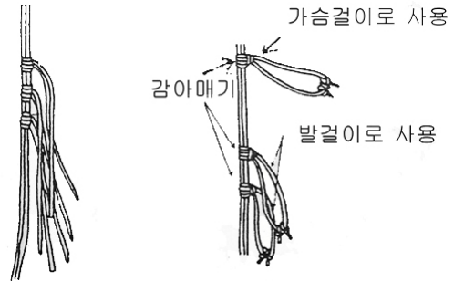
(그림 3-91) 감아매기 등반 로프 만들기
