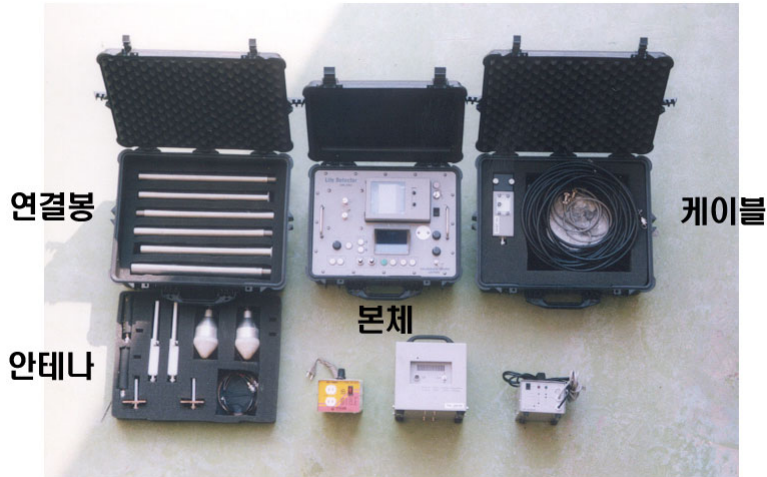
(그림 2-18) 매몰자전파탐지기
