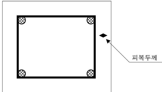
(그림 5-88) 철근 콘크리트 기둥의 단면도
