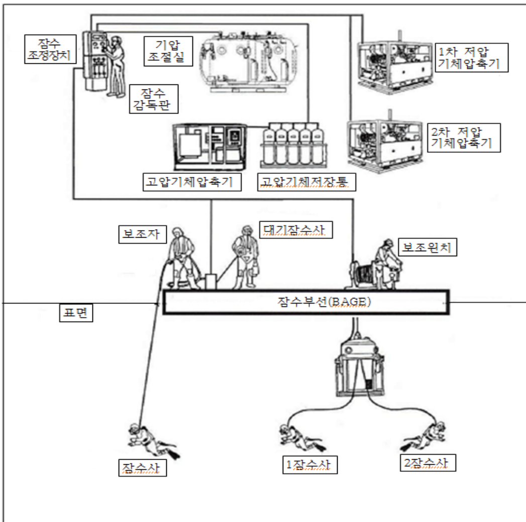
(그림 5-82) 표면공급식 잠수운영 계획도
