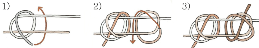
(그림 3-18) 이중피셔맨매듭
