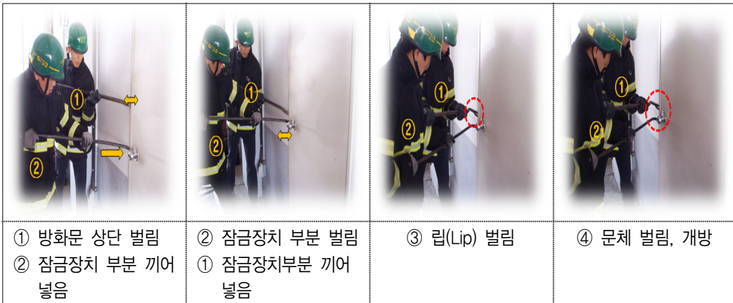
(그림 6-26) 2인1조 지렛대(배척) 활용 작업
