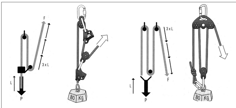
(그림 2-29) 도르래 설치방법의 예
