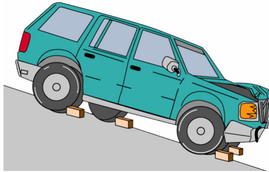
(그림 5-19) 경사면에 주차된 차량의 고임목
