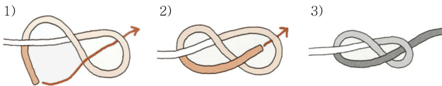
(그림 3-4) 8자매듭
