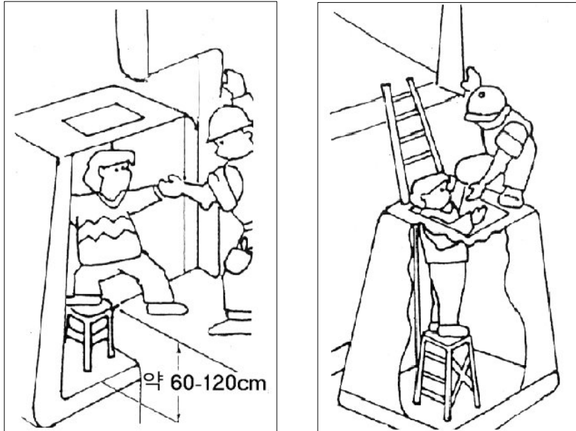
(그림 5-107) 승장과 카의 높이 차이가 60cm 이상인 경우에는 외부의 도움을 받아야 한다.
