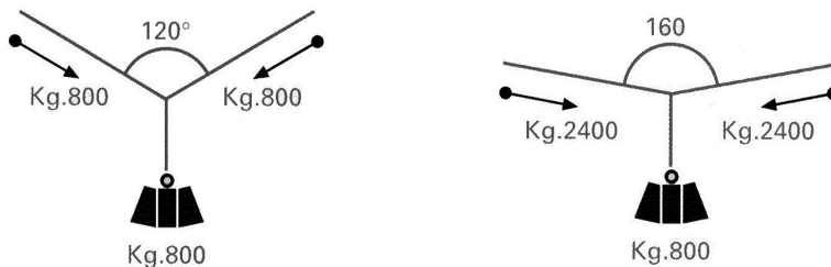
(그림 3-55) 수평으로 연장된 로프에 가해지는 장력
