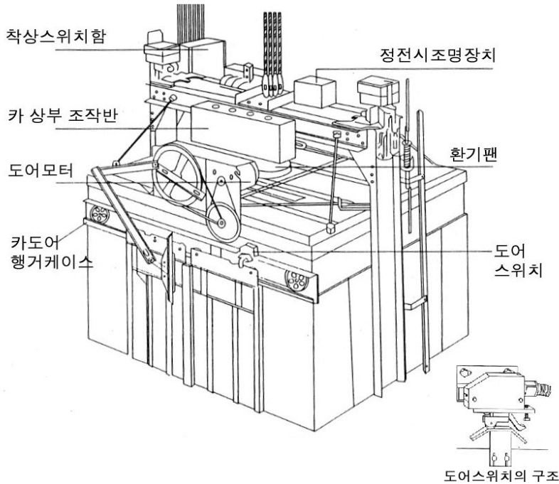
(그림 5-104) 카 상부의 구조
