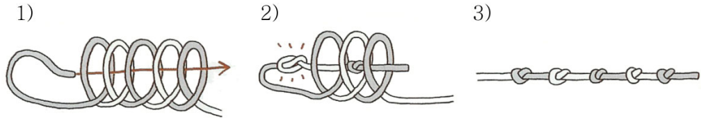
(그림 3-8) 줄사다리매듭
