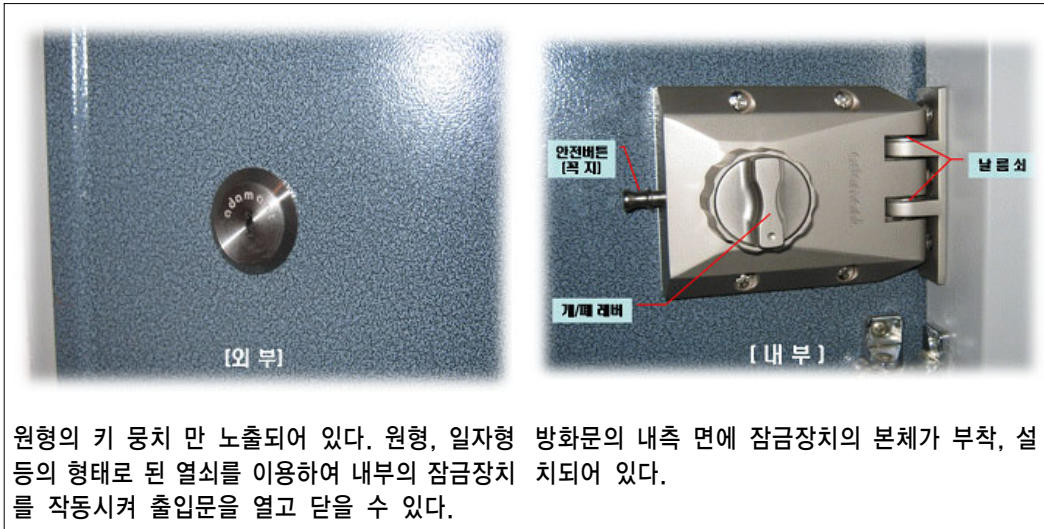
(그림 6-4) 보조 잠금장치
