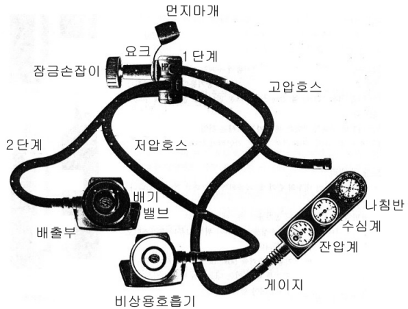
(그림 5-70) 호흡기(Regulator)
