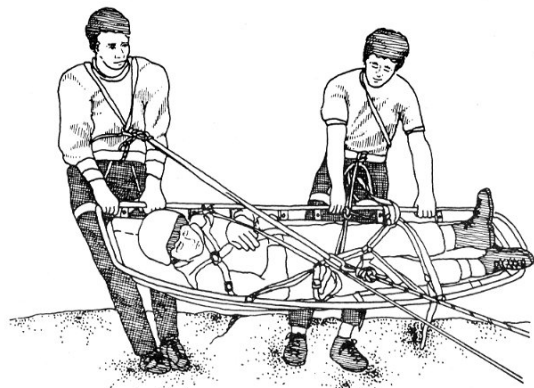
(그림 5-116) 1줄 로프로 하강하기
