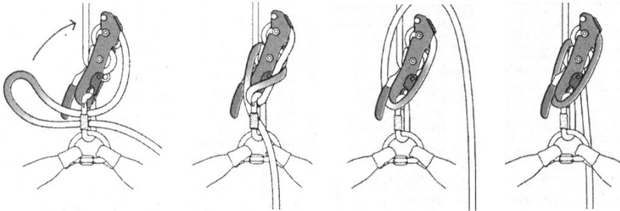
(그림 3-81) 스톱하강기 고정법
