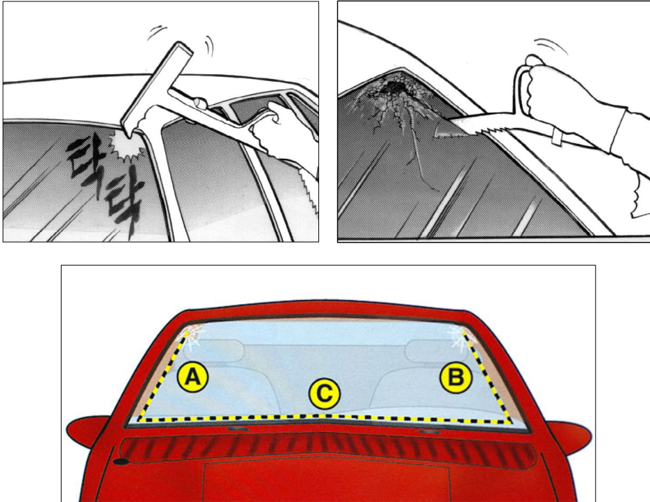
(그림 5-28) 앞 유리는 A,B 지점을 타격한 후 U자 형태로 잘라낸다.
