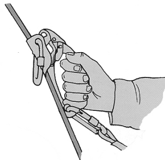
(그림 3-86) 로프가 이탈하지 않도록 카라비나를 끼워둔다.
