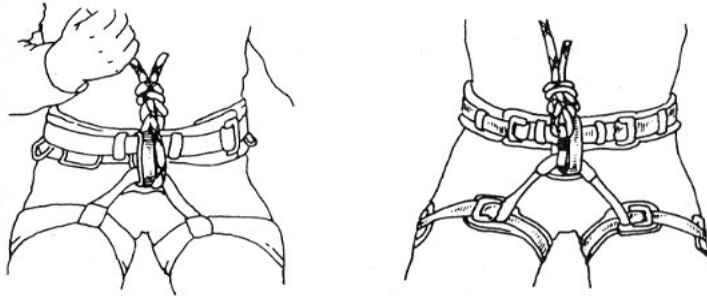
(그림 5-111) 안전벨트에 로프를 묶는 법
