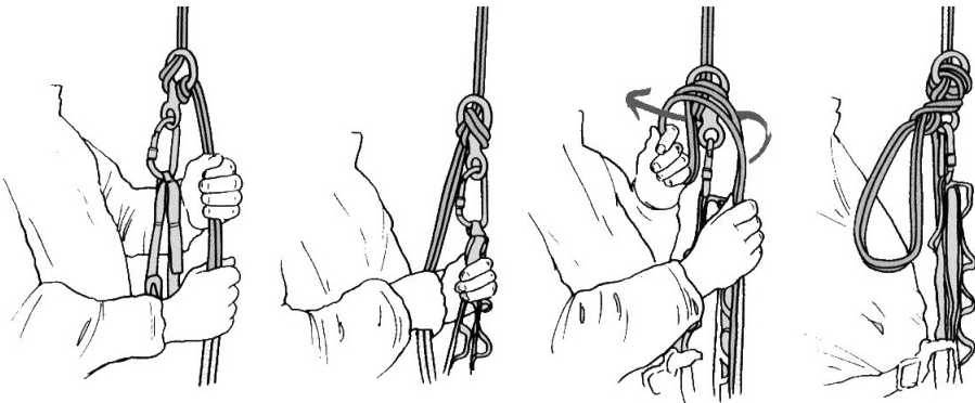
(그림 3-79) 8자 하강기를 완전히 고정하는 방법
