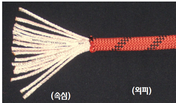
(그림 2-19) 컨먼틀 로프의 구조
