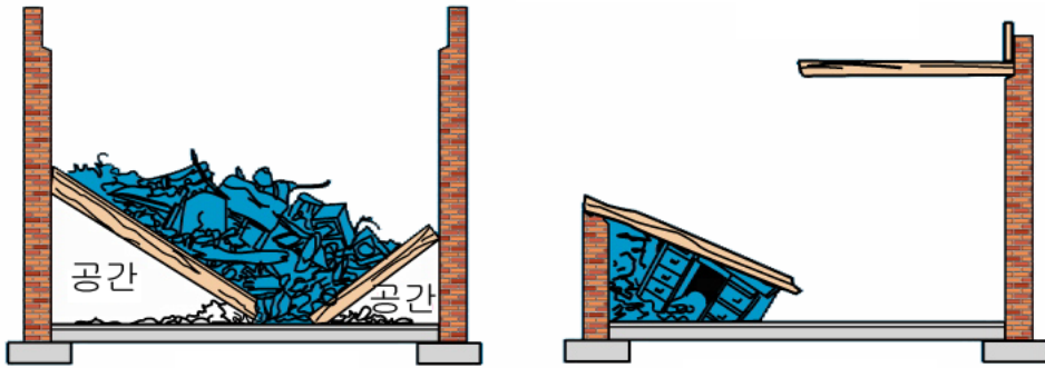
(그림 5-92) V자형 붕괴(좌)와 캔틸레버형 붕괴
