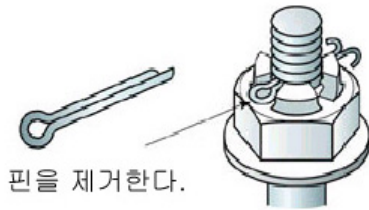
(그림 5-11) 고정핀을 제거한다.
