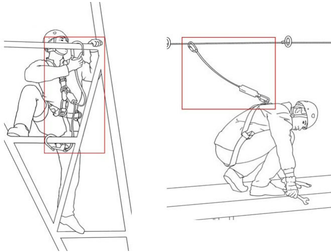
(그림 3-65) 자기확보 취하기
