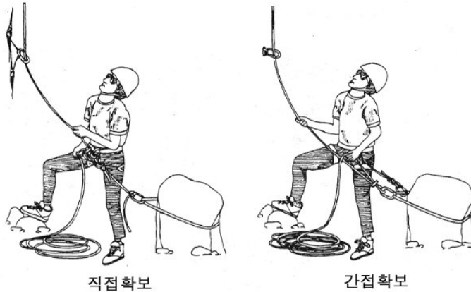
(그림 3-63) 직접확보와 간접확보
