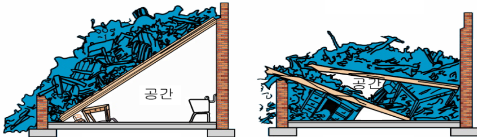
(그림 5-91) 경사형 붕괴(좌)와 팬케이크 붕괴(우)
