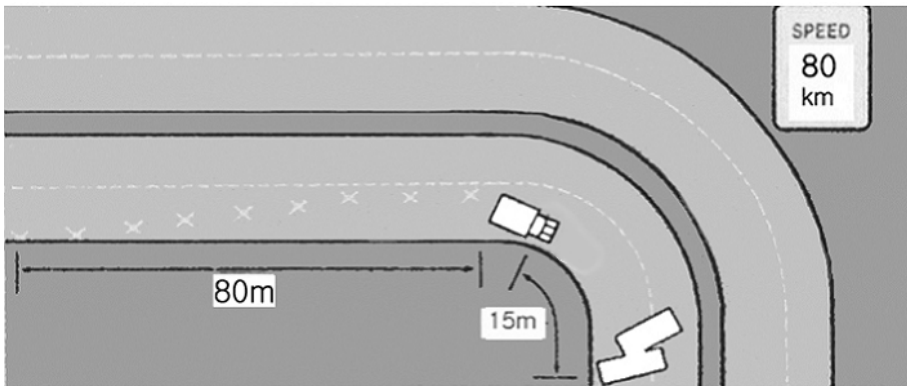
(그림 5-16) 곡선도로에서 사고가 발생한 경우 곡선 시작부분에 주차하고 후방으로 80m 이상 유도표지를 설치한다.
