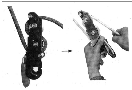
(그림 2-24) 스톱 하강기 사용법
