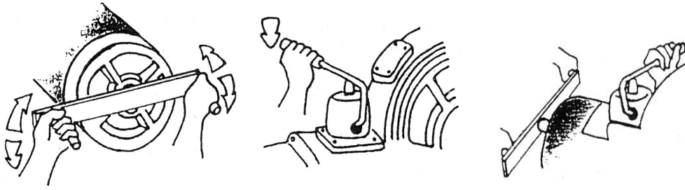
(그림 5-108) 터닝 핸들과 브레이크의 조작방법 브레이크는 슈브 반대쪽에서 개방한다.
