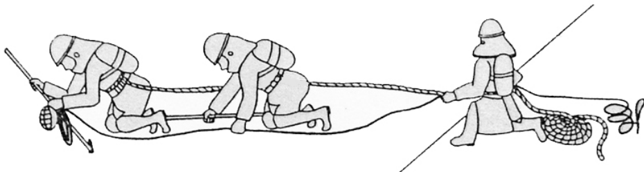
(그림 4-38) 농연 속에서는 자세를 낮추고 진입한다. 선 진입자에게 유도로프를 결착하여 후진입자가 이를 잡고 진입할 수 있도록 한다.
