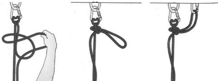
(그림 3-51) 카라비나에 로프 결착하기
