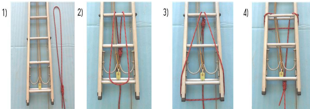
(그림 3-30) 사다리 묶기
