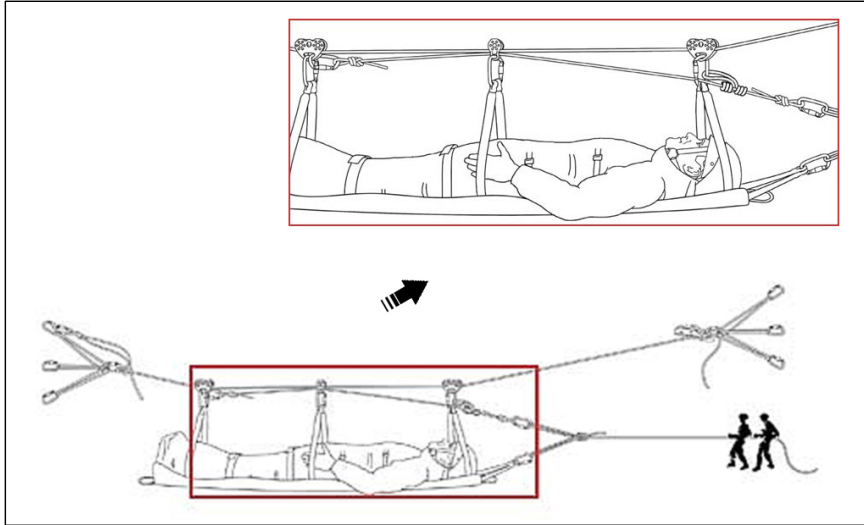
(그림 4-25) 들것을 이용한 요구조자의 구출
